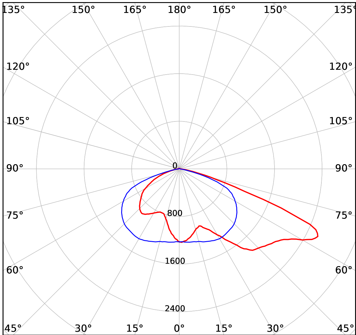
cd 6000 lm — C0-C180 — C90-C270
