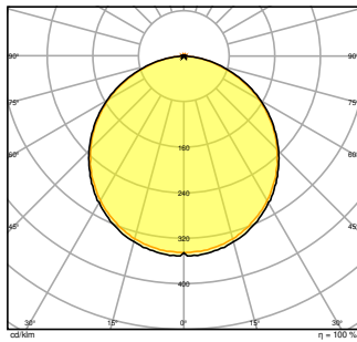
PL CMFT 600 P 33W 830 PS EM CONVERSION BOX
