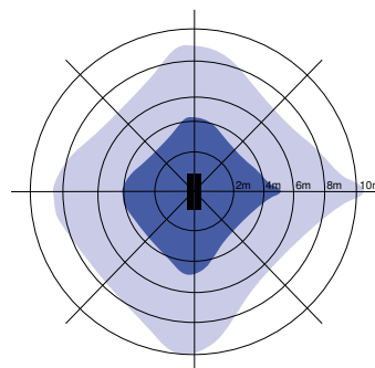
Installatie - Middel plafond Aanbevolen installatie hoogte 12m
