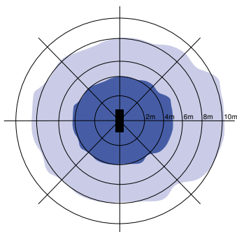
Installatie - Laag plafond Aanbevolen installatie hoogte 9m
