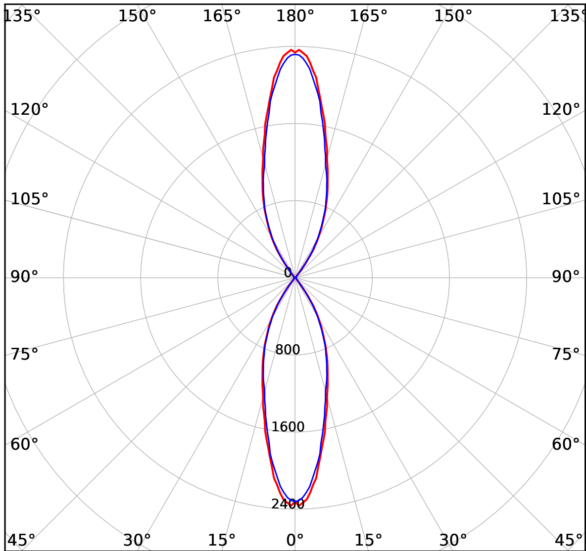
cd 2100 lm — C0-C180 — C90-C270
