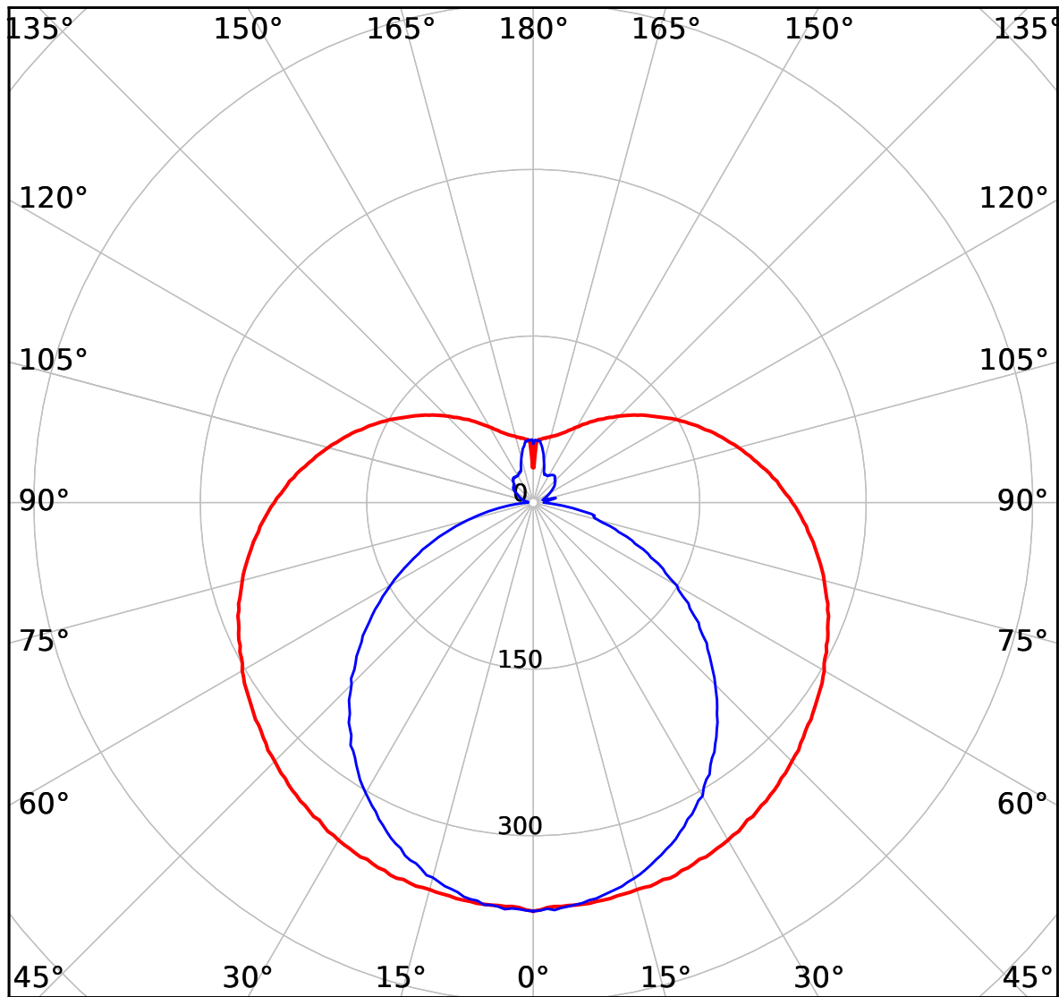
cd 2000 lm — C0-C180 — C90-C270
