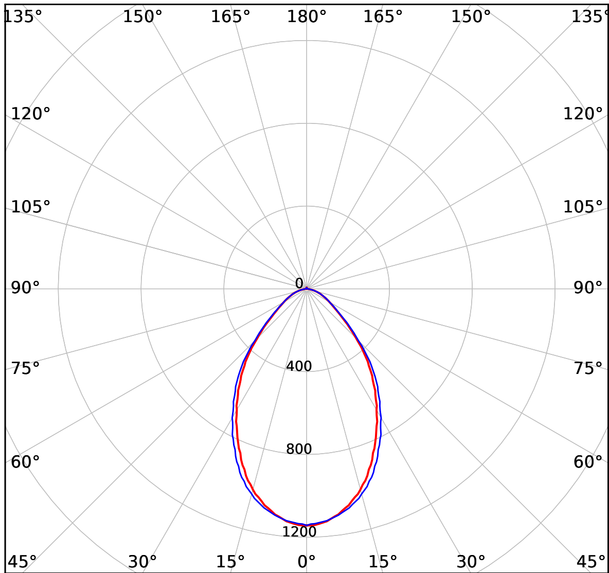
cd 1725 lm — C0-C180 — C90-C270
