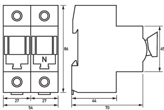
Maßzeichnung Gruppenansicht
