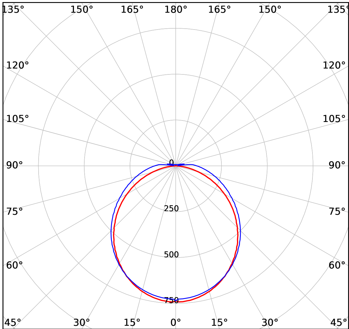
cd 2300 lm — C0-C180 — C90-C270
