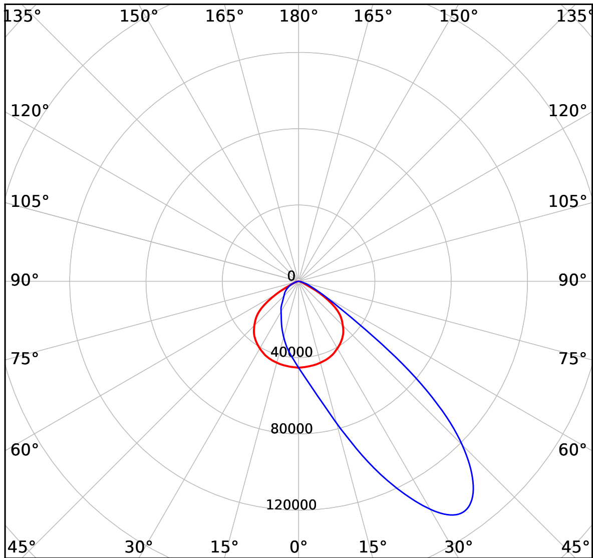
cd 150000 lm — C0-C180 — C90-C270
