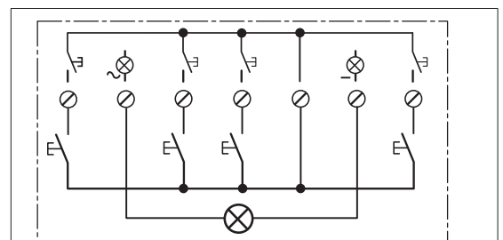
art. 2141 - 043 650 2142 - 043 653 2143 - 043 626 2144 - 043 659
