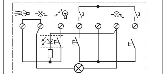
art. 2130 - 043 621 2131 - 043 624 2132 - 043 627
